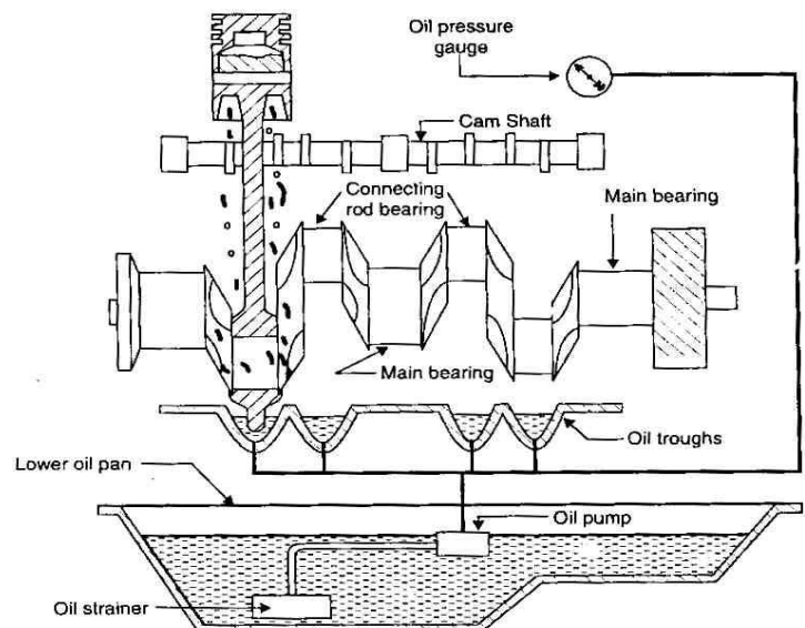
Fig. 4.23. Splash system.
